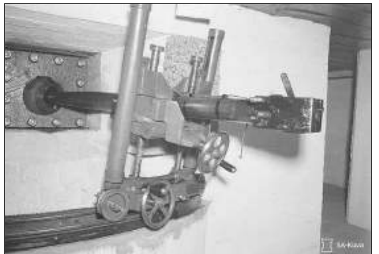
45mm tykki korsussa Virolahden Ravijoella 11.4.1941.
