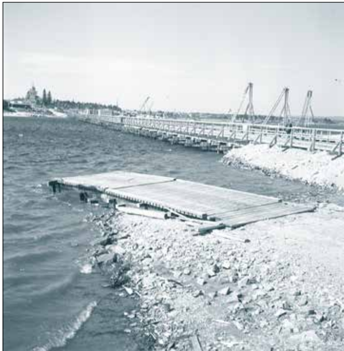
Saksalaisten pioneerien rakentama tilapäissilta Kemijärven yli. Rakennusaika oli 7-8 päivää. Työssä 700-800 miestä. Kemijärvi 14.7.1941.
