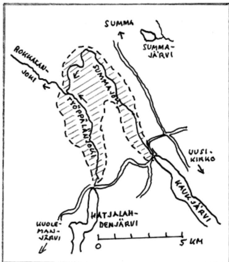
Rokkalanjoen suulle ja Hatjalahdenjärven pohjoispäähän rakennetut padot sulkemalla saatiin Summa- ja Työppälänjokilaaksot veden valtaan. Piirroksen on merkitty vinoviivituksella alue jonka tulva korkeimmillaan peittäisi.
