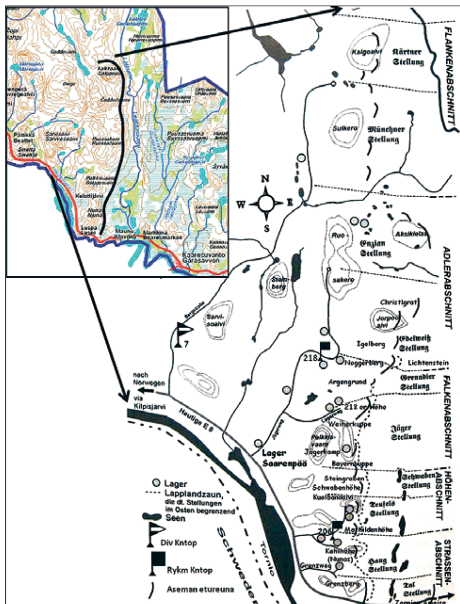
Sturmbock-aseman rakenne, sijainti Lätäsenon länsipuolella ja saksalaisten käyttämä ”täydennetty” maaston nimikkeistö. Nykyinen Järämän museo sijoittuu paikkaan, jossa alareunan ”Grenzbergin” asema leikkaa Käsivarren tien (nyk. E8). Lähde: DAWA Stellungsskizze, osa nimistöä ja ryhmitys kirjoittajan.
