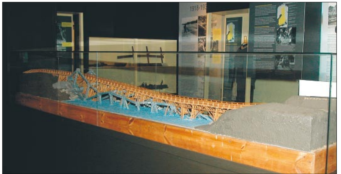
Yksi sisätilan näyttelyn uljaimmista nähtävyyksistä on Kiviniemensillan pienoismalli. Sillan pituus oli 105 m ja kantavuus 7 tonnia, joka hyvin riitti sen aikaisten ajoneuvojen painolle. Silta oli käytössä talvisodan aikana ja jatkosodan alkaessa, mutta purettiin 1942. Samalle paikalle rakennettiin rautatiesilta 1942-43, joka räjäytettiin vetäytymisvaiheessa 1944.
